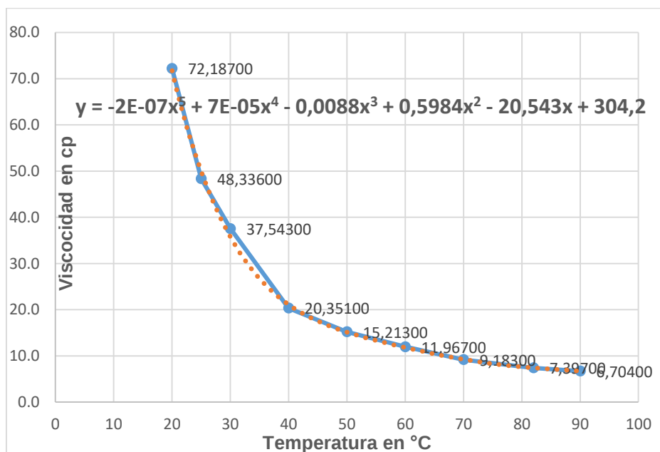
Figura 3. Perfil de viscosidad de aceite de calabaza en relación de temperatura.
